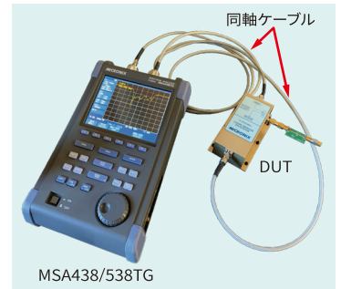
図1.接続の仕方
