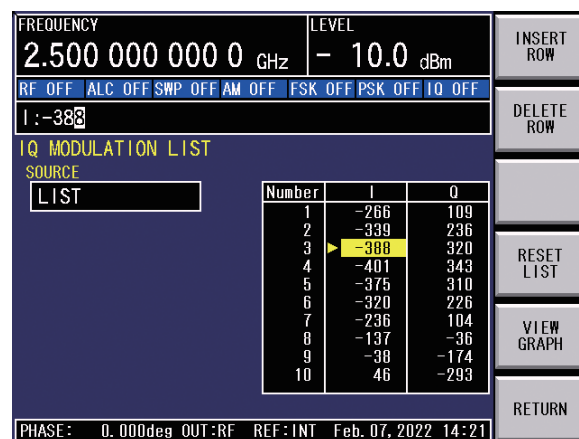
リストデータ編集画面
