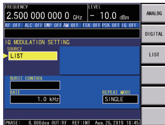
リストデータ設定画面
