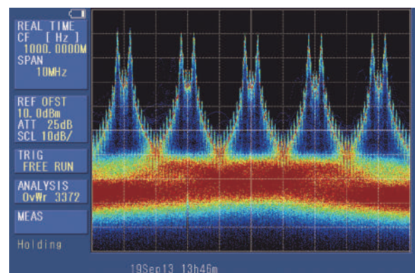
シグナルアナライザMSA538のオーバーレイ画面
