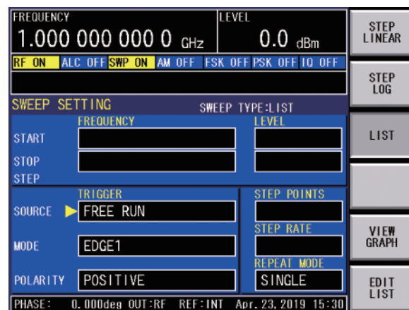
リスト掃引設定画面
