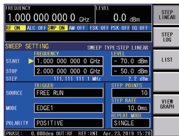
ステップ掃引設定画面
