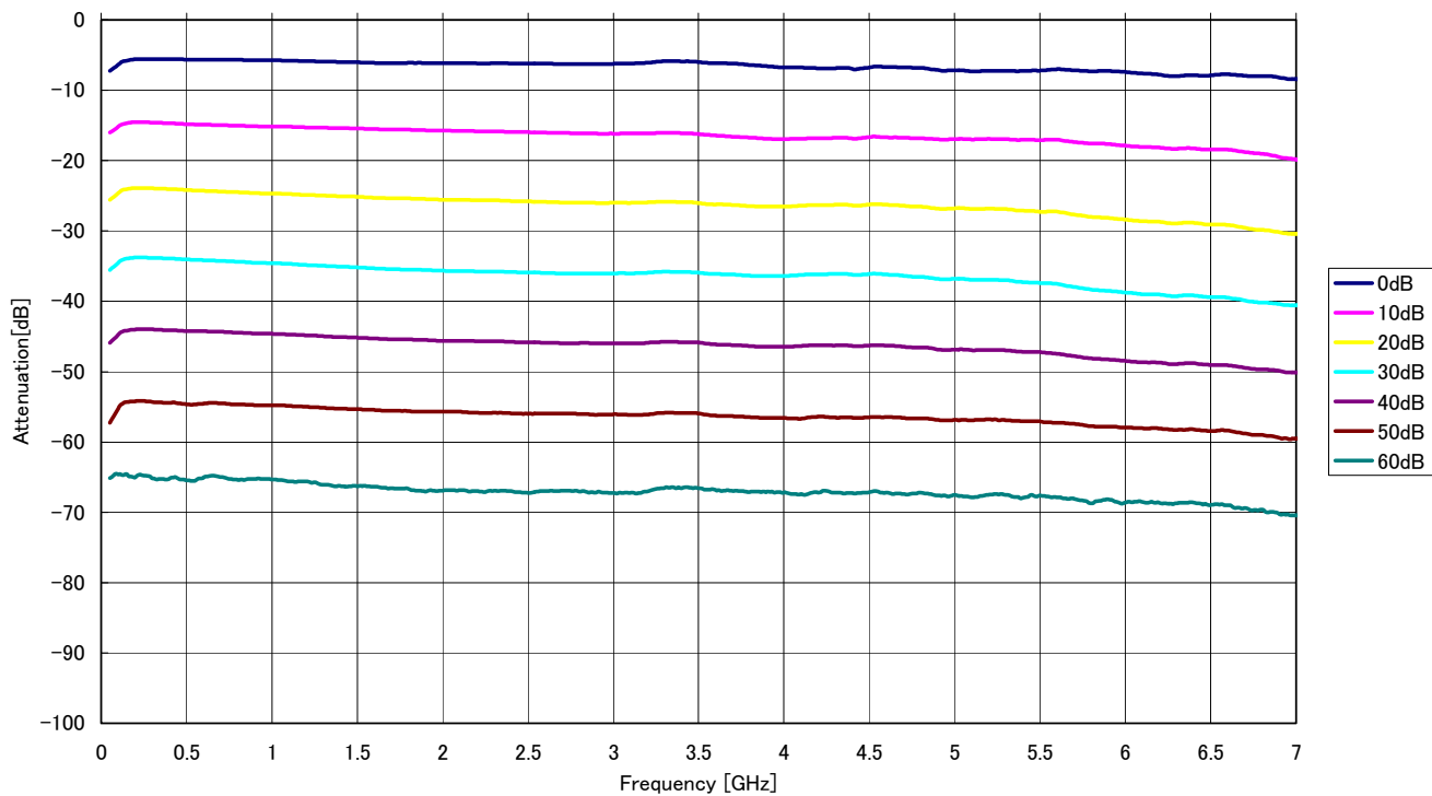
MAT850 Attenuation(S21)
