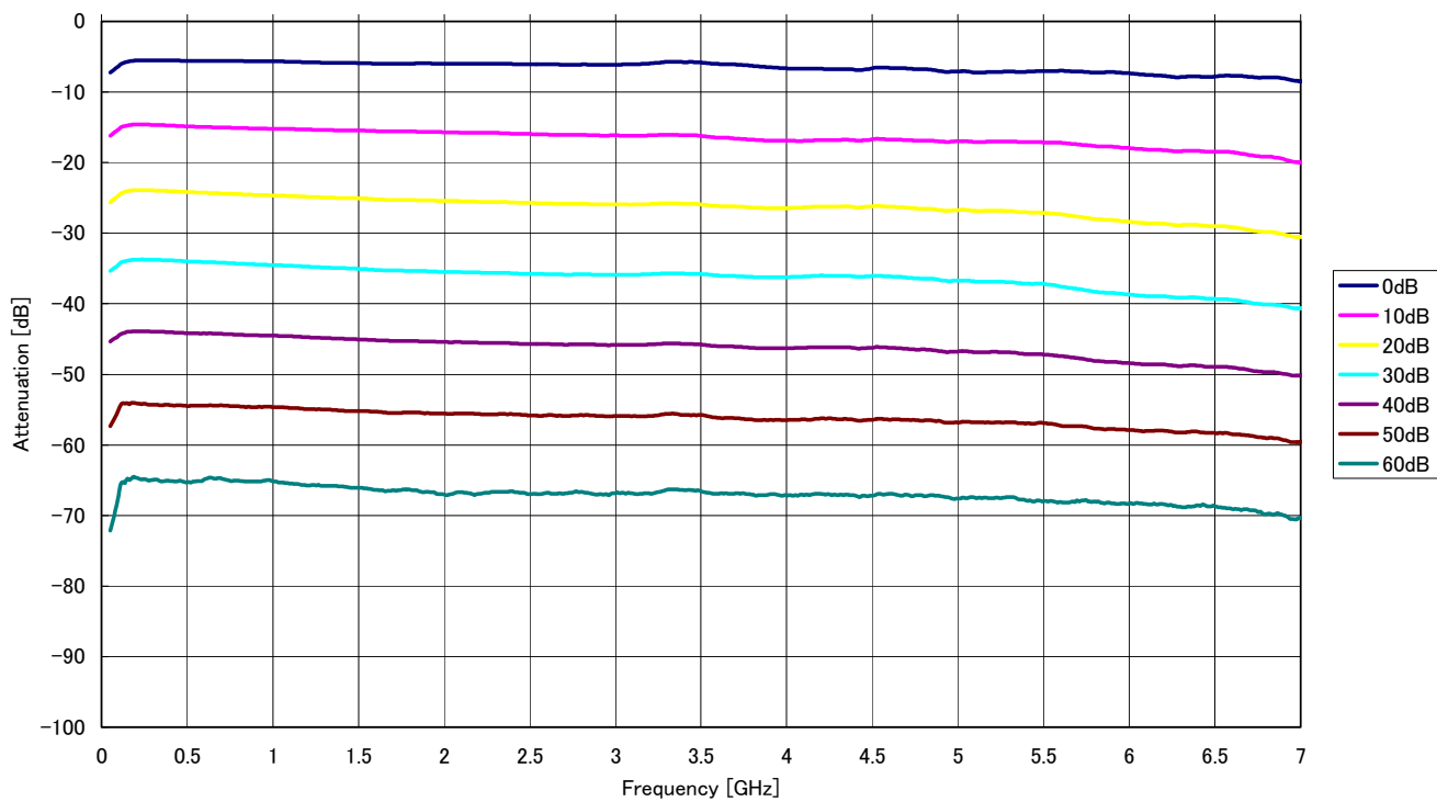
MAT850 Attenuation(S21)
