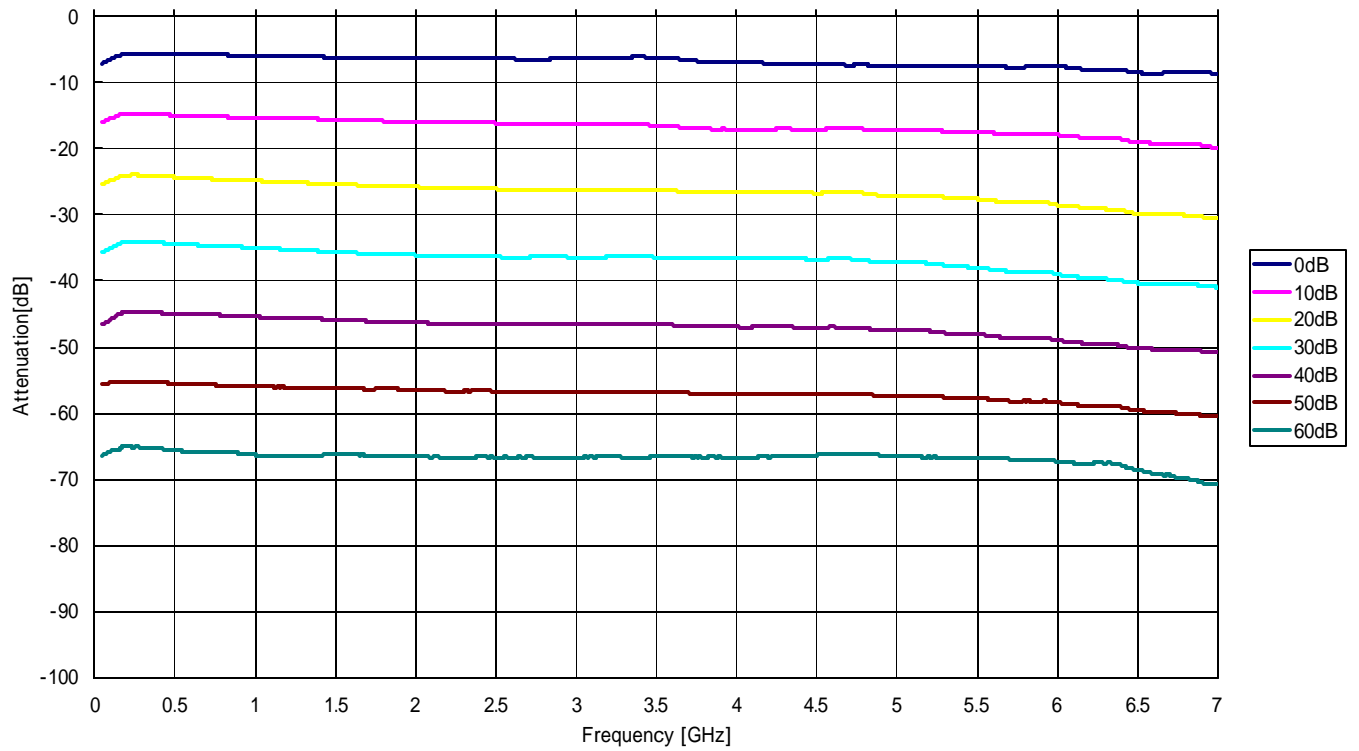
MAT810 Attenuation(S21)
